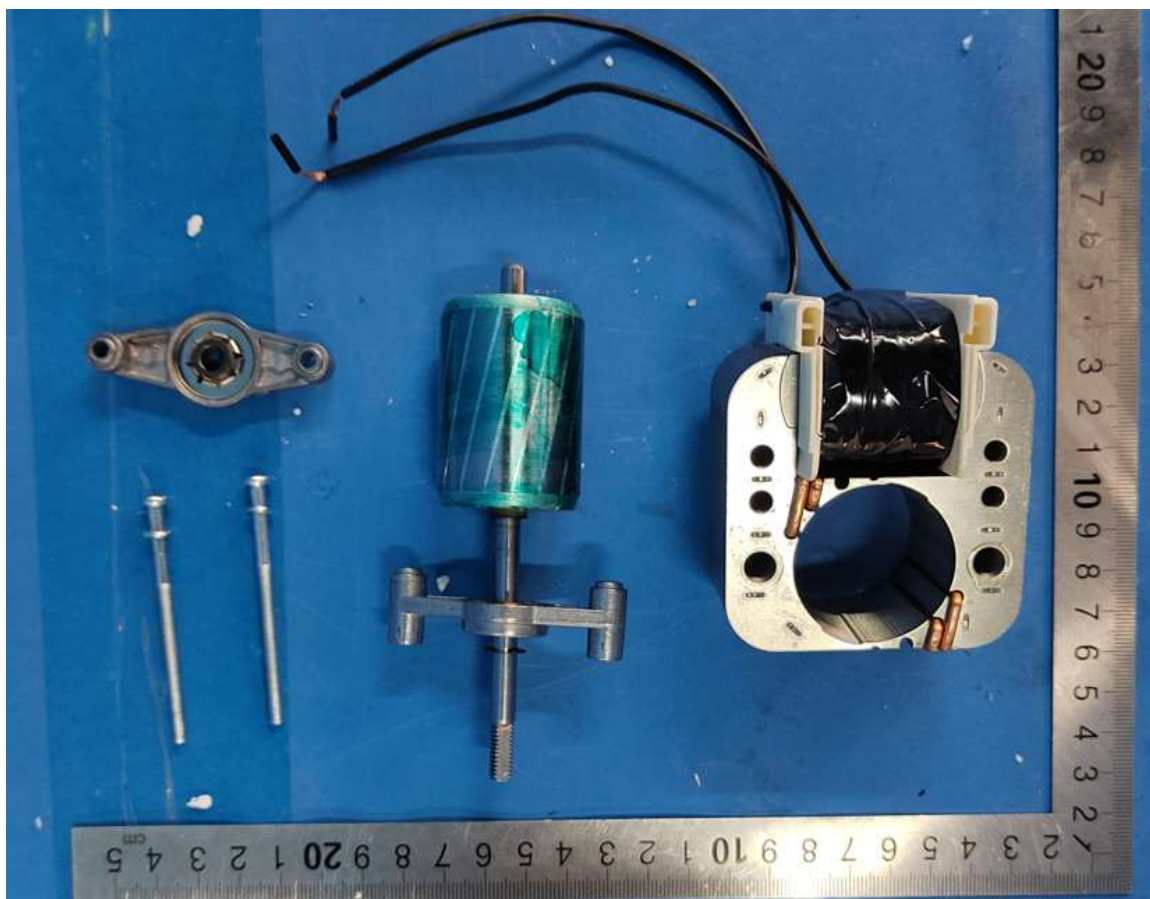
S60B-A13-LX 内部结构
