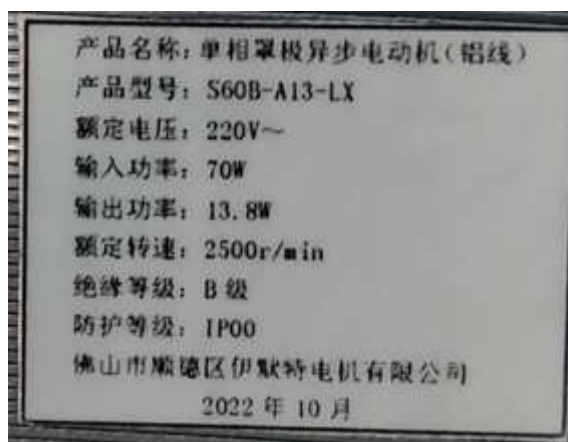
铭牌(材质: 哑银不干胶)
