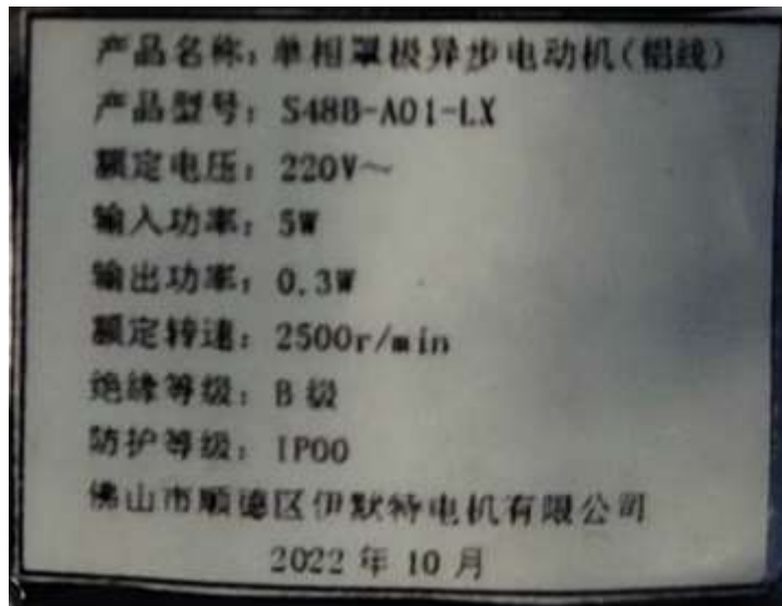
铭牌(材料: 哑银不干胶)
