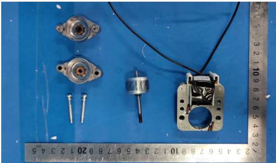
S48B-A01-LX 内部结构
